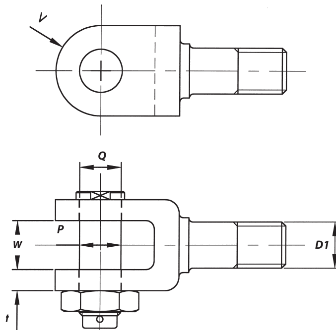
Jaw (double lug) head fittings DIN 82008 / ISO 6043
